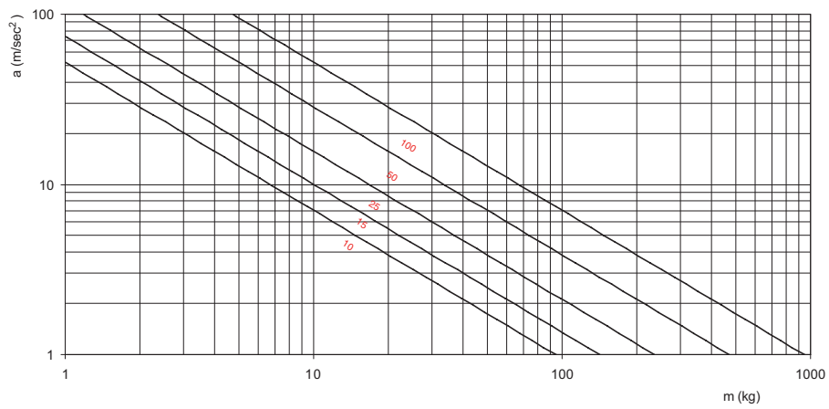
HTD5M
