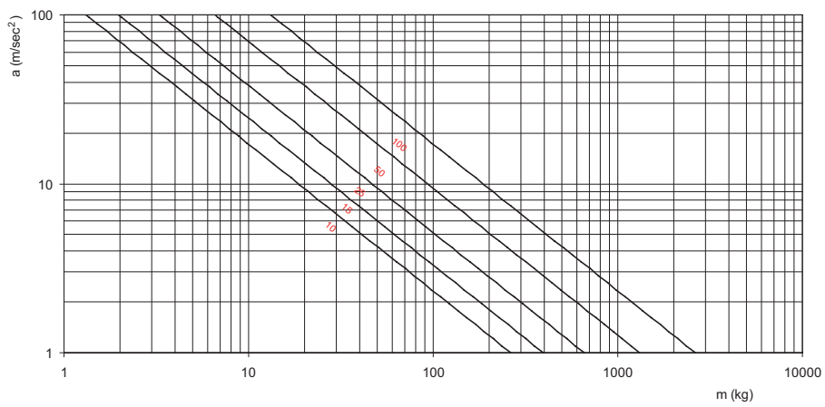
HTD8M
